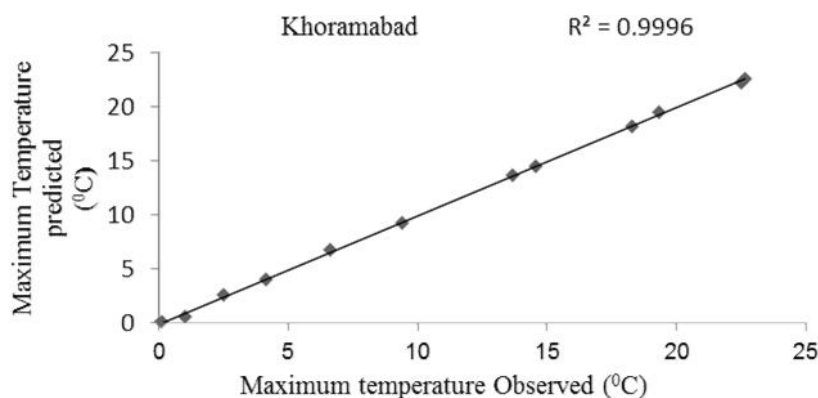
شکل ۲- ضریب تعیین حداکثر دمای مشاهداتی و پیش‌بینی شده ایستگاه در خرم‌آباد (۱۹۸۰-۲۰۱۰ و ۲۰۱۱-۲۰۳۰)
