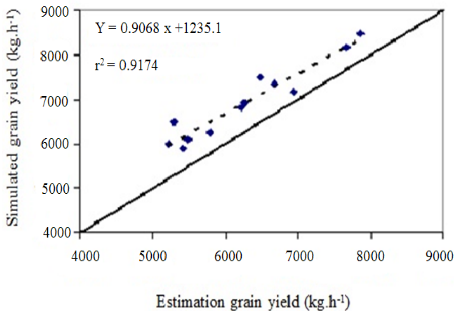
شکل ۱- مقایسه بین عملکرد دانه شبیه سازی شده و مشاهده شده گندم Fig. 1- Comparison between simulated and estimated wheat grain yields
